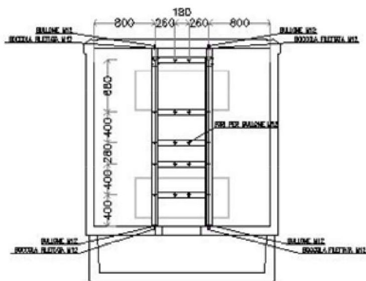
SEZIONE D1 - D1
