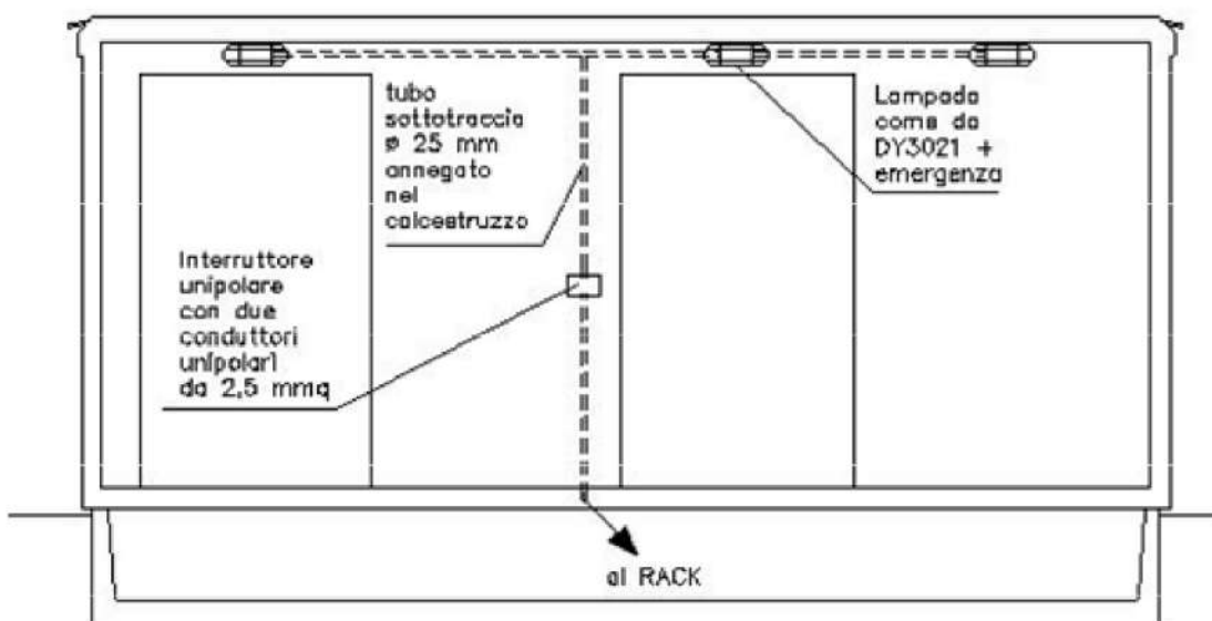
SEZIONE C1 - C1
