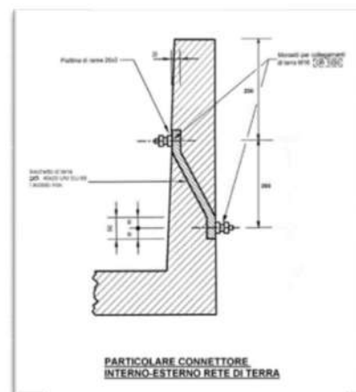
Connettore interno/esterno per rete di terra
