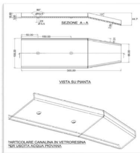
Canaletta uscita acqua piovana
