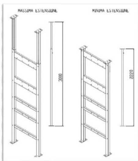
Telaio porta quadri BT
