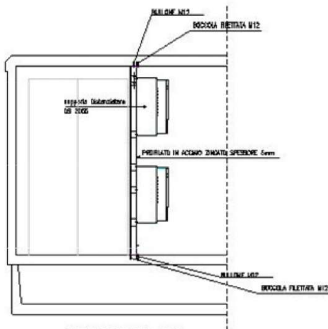
SEZIONE D2 - D2
