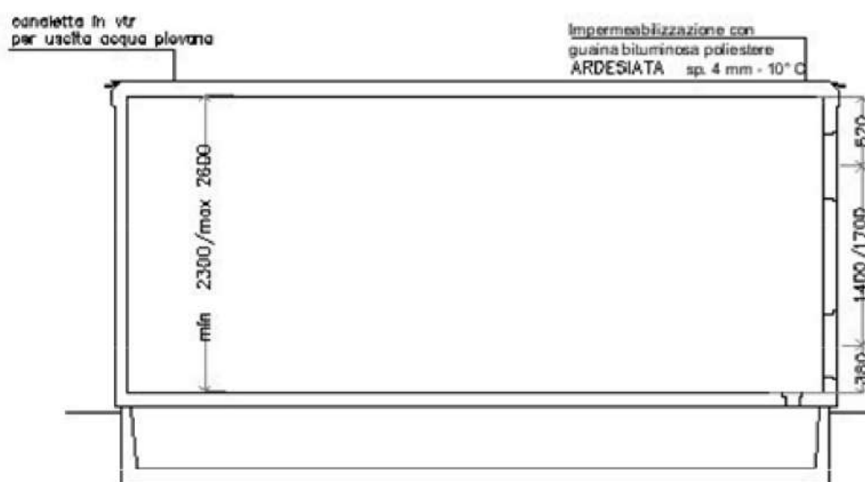
SEZIONE C - C
